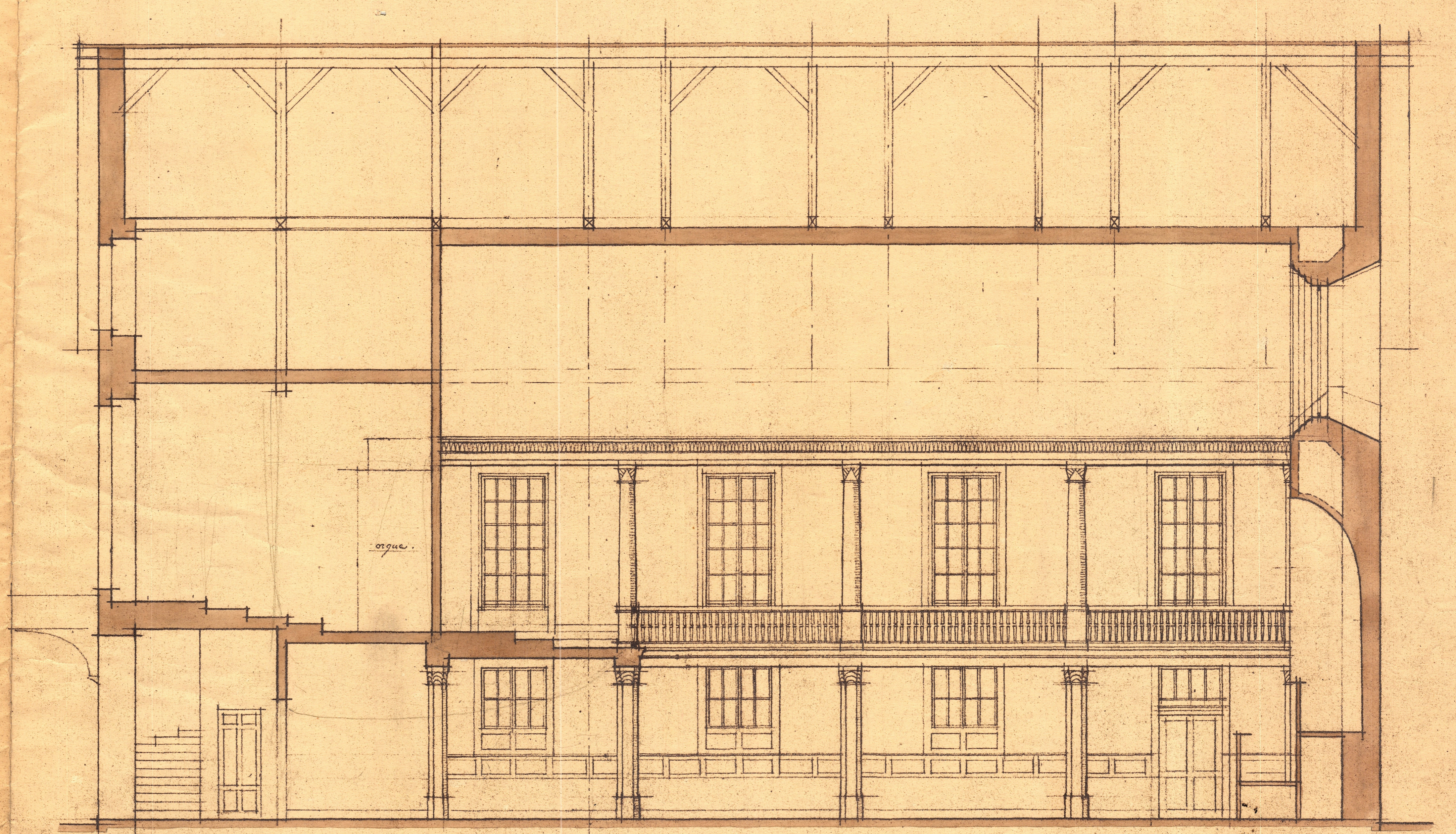
COUPE LONGITUDINALE
