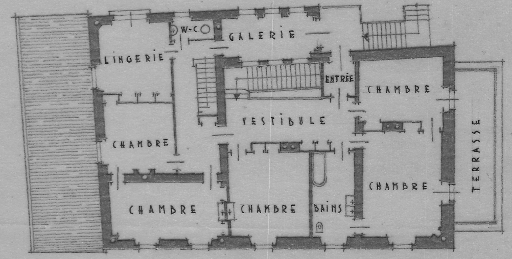
1 ER ÉTAGE
