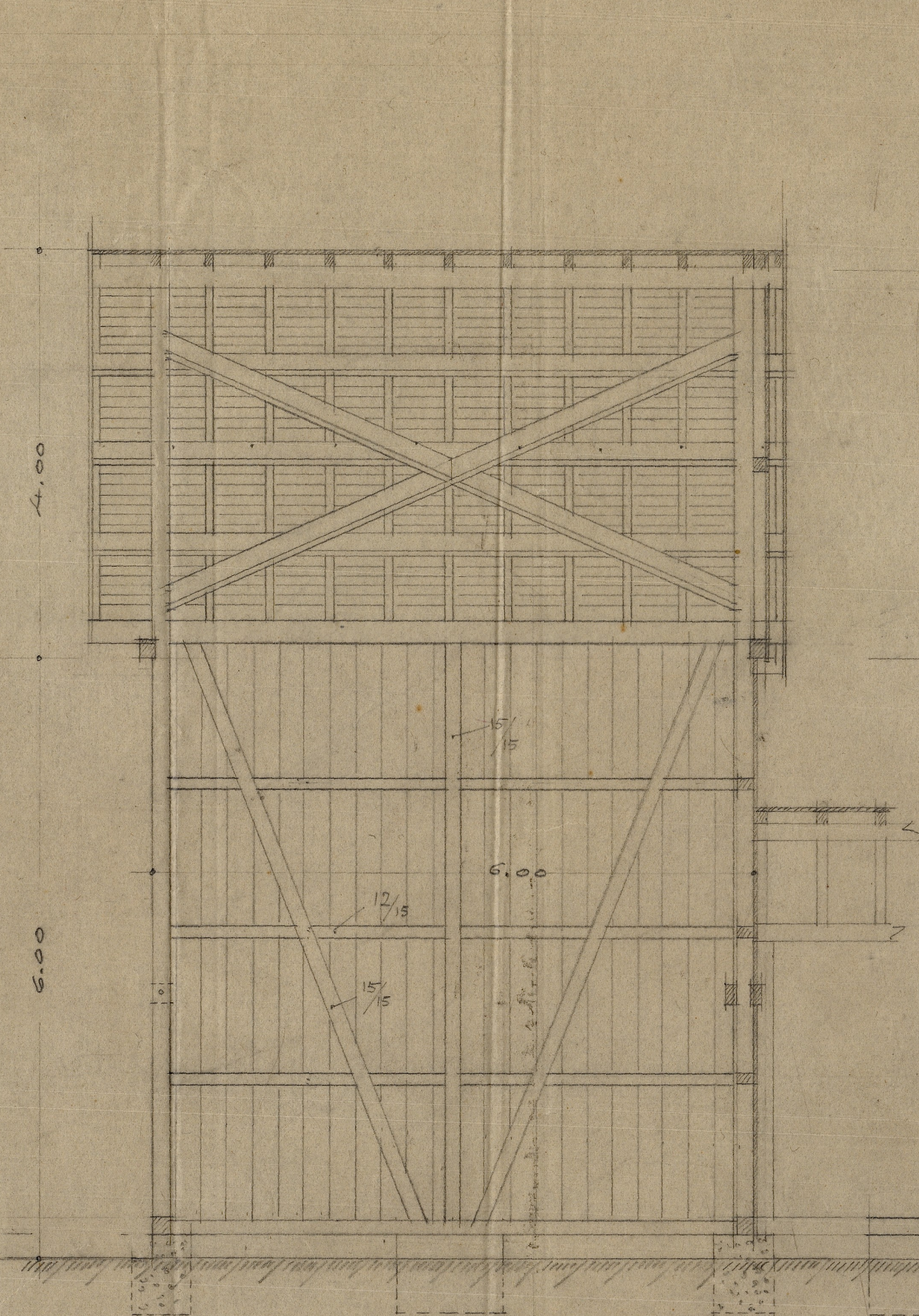
COUPE LONGITUDINALE
