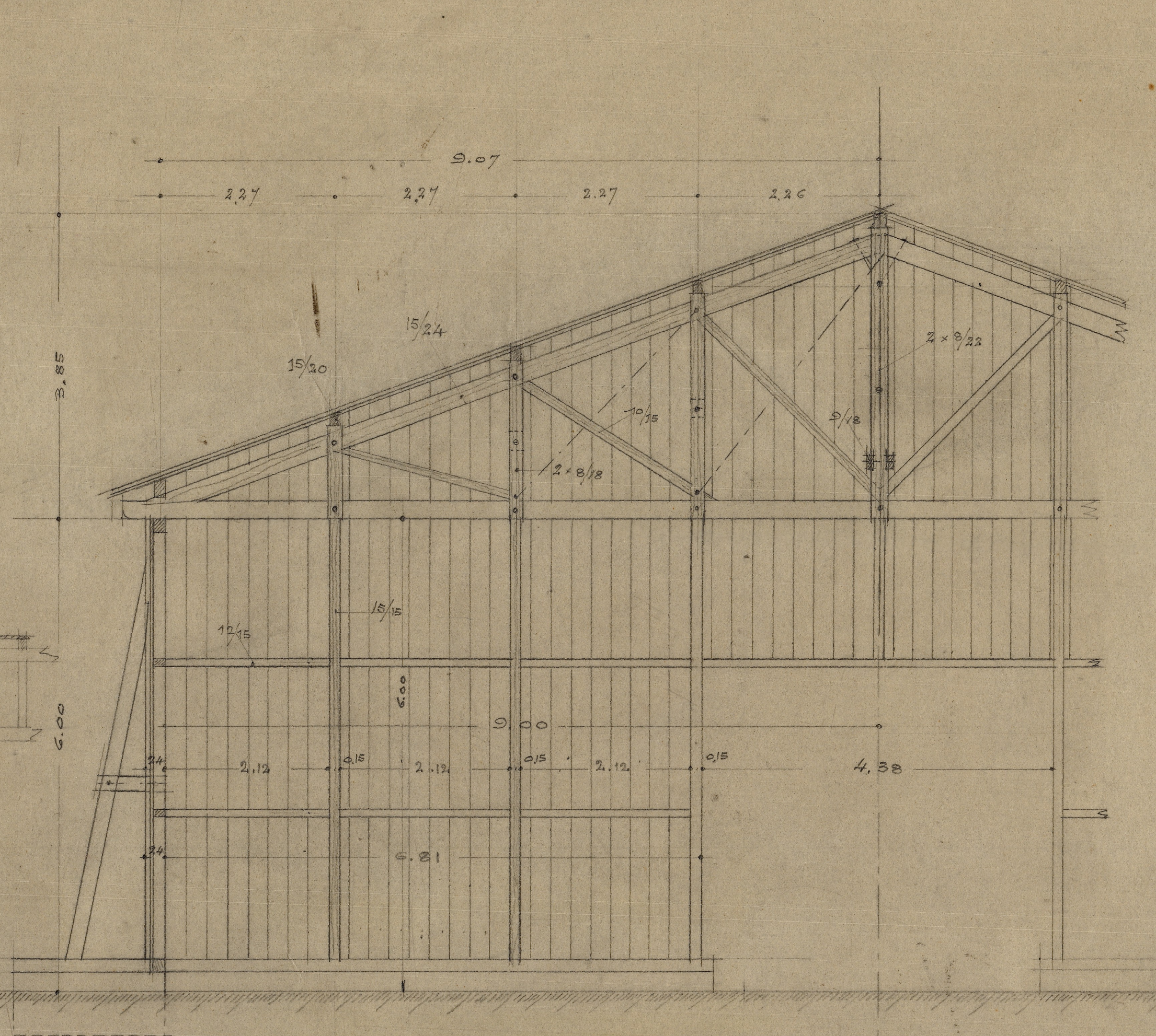
COUPE VARIANTE
